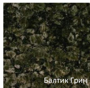
Сопка Бунтина
